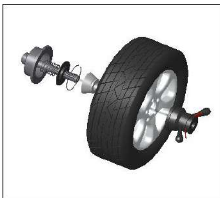
конус «внутри» (на быстрозажимную гайку нужно установить прижимную чашку)
